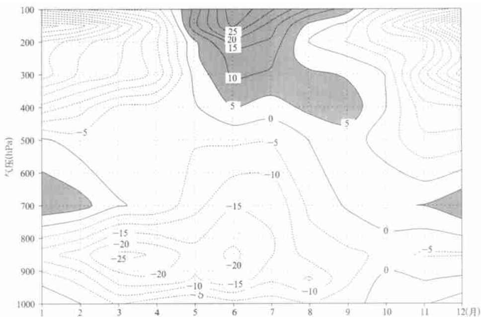
图 7 用探空资料计算出的高原以东地区(25 ~ 35°N, 103 ~ 120°E) 1990 ~ 1998 年累年平均散度的季节变化(单位: 10^{-7}/s )
