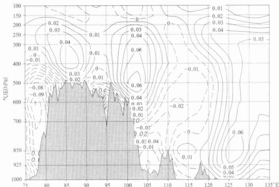
图 6 1979 ~ 1996 年累年平均 2 月份沿 30°N 垂直速度的高度-经度分布(NCEP 资料,单位: Pa/s)
