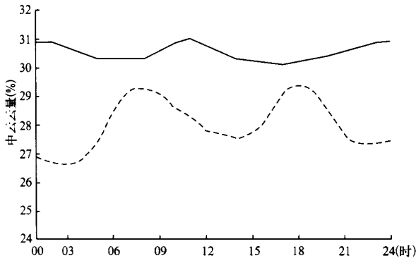
图 12 高原以东地区(25~35°N, 103~120°E)卫星中云云量和地面观测中云云量的日变化(实线为 ISCCP1990~1998 累年平均中云量的日变化,虚线为 2001 年 30 个站点平均的年平均中云量的日变化)
