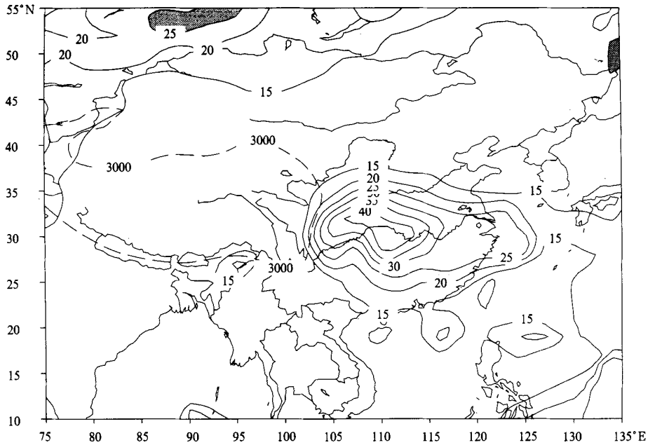
图3 1990~1998年中国及周边部分地区(10~55°N,75~135°E)地面观测2月份中云云量累年平均分布
