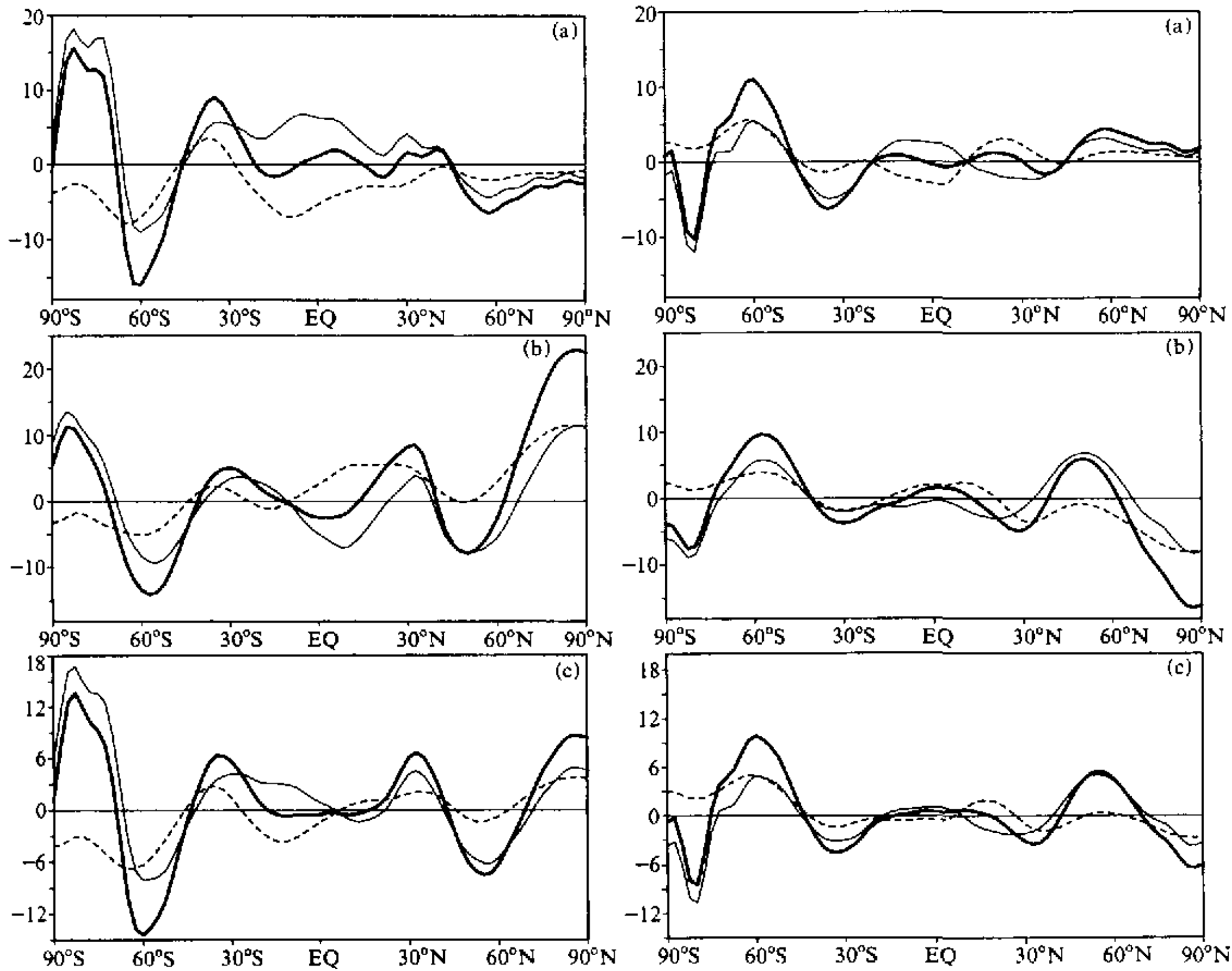
图 12 1958~1997 年 30^{\circ}\text{E}\sim 80^{\circ}\text{E} 区域内平均指数 (\bar{I})_{\text{E}} (粗实线)、 (\bar{I}_1)_{\text{E}} (虚线) 和 (\bar{I}_2)_{\text{E}} (细实线) 的经向廓线分布 (单位: 10^3 \text{ kg m}^{-1} \text{ s}^{-1} ) (a) 夏季; (b) 冬季; (c) 年平均
