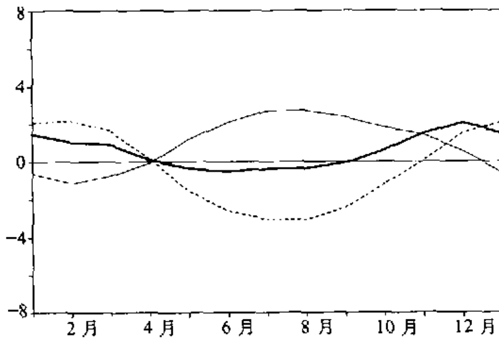
图14 1958~1997年赤道圈上 177.5^{\circ}\text{W}\sim 27.5^{\circ}\text{E} 区域内平均的指数 (\bar{I})_w (粗实线), (\bar{I}_1)_w (虚线)和 (\bar{I}_2)_w (细实线)的年变化(单位: 10^3 \text{ kg m}^{-1} \text{ s}^{-1} )
