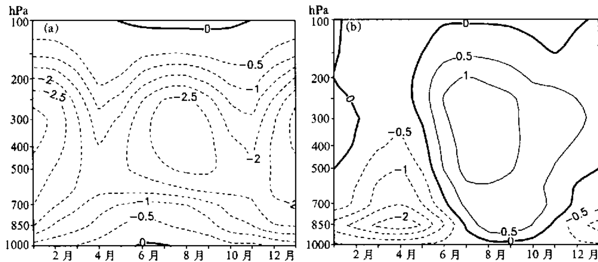
图 15 1958~1997 年赤道上区域平均垂直速度 \bar{\omega} 的月份-高度剖面图 (单位: 10^{-4} \text{ hPa s}^{-1} ) (a) 30^{\circ}\text{E} \sim 180^{\circ}\text{E} ; (b) 177.5^{\circ}\text{W} \sim 27.5^{\circ}\text{E}
