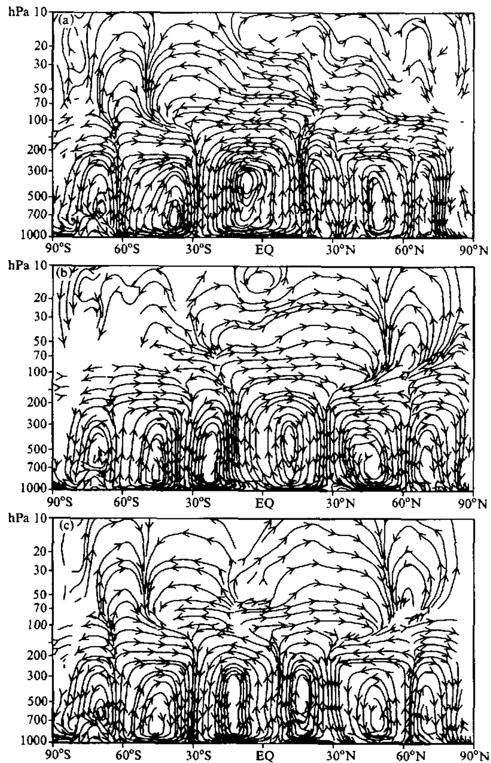
图6 1958~1997年纬向平均经圈环流 [\bar{C}_{yz}] 的流线图 (a) 夏季 (JJA); (b) 冬季 (DJF); (c) 年平均
