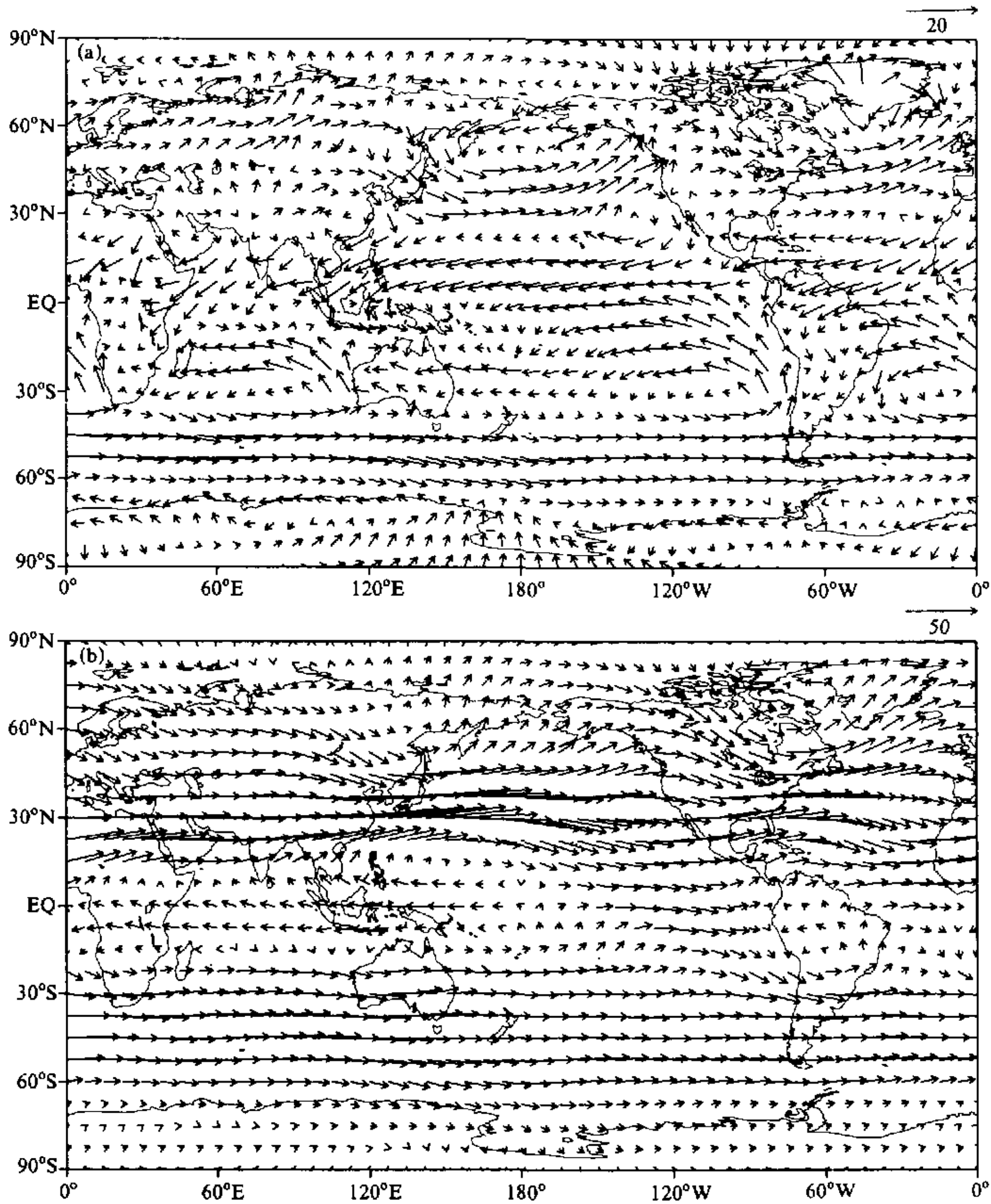
图2 同图1, 但为冬季(12、1、2月, 即DJF)
