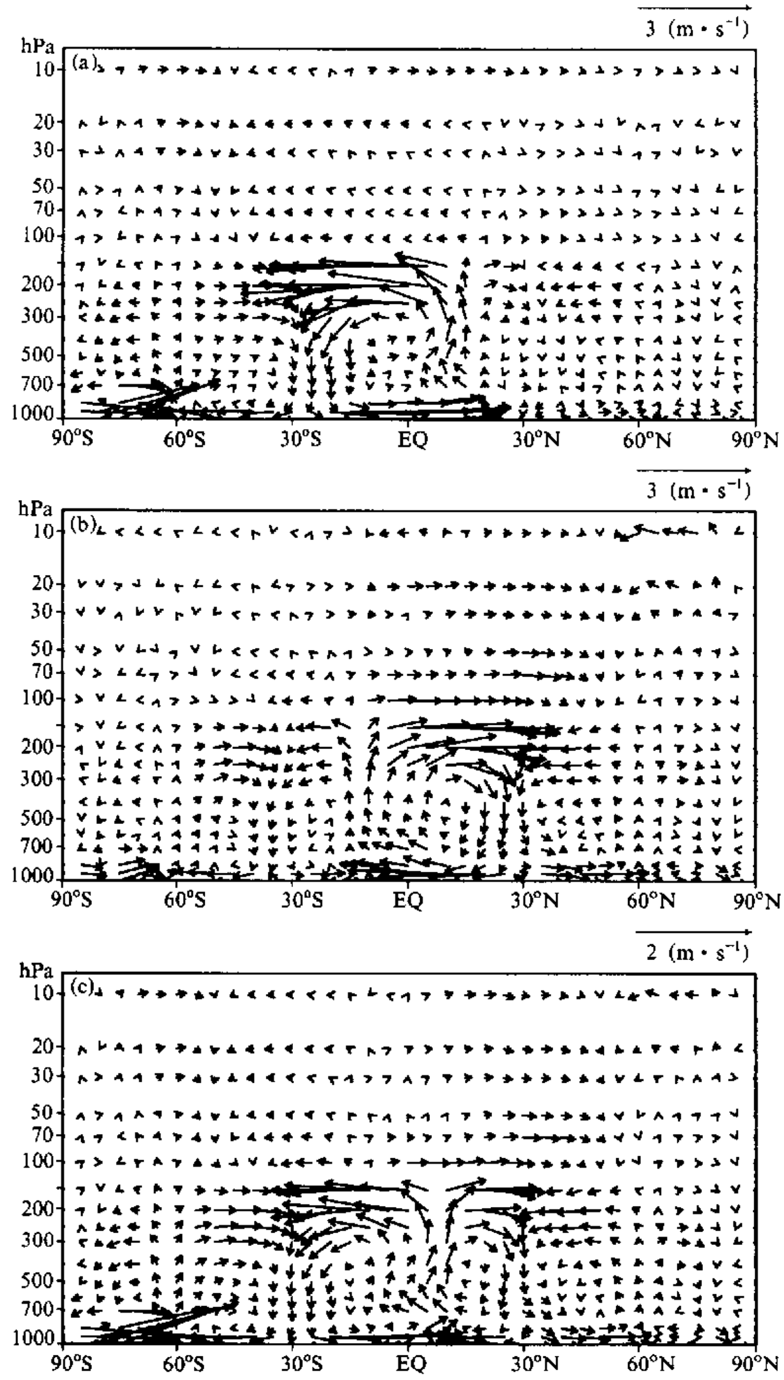
图 5 1958~1997 年平均经圈环流 \overline{C}_{\text{mer}} 图 (a) 夏季 (JJA); (b) 冬季 (DJF); (c) 年平均
