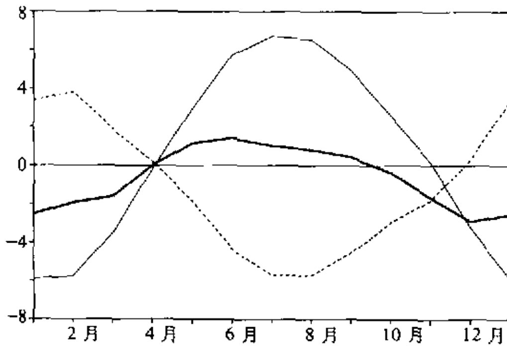
图 11 1958~1997 年赤道圈上 30\sim 180^\circ\text{E} 区域内平均的指数 (\bar{I})_E (粗实线)、 (\bar{I}_1)_E (虚线) 和 (\bar{I}_2)_E (细实线) 的年变化 (单位: 10^3 \text{ kg m}^{-1} \text{ s}^{-1} )
