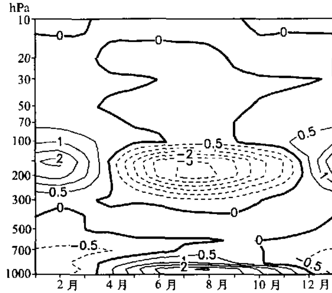
图4 1958~1997年赤道上沿纬圈平均经向风 \bar{v} 的月份-高度剖面图(单位: \text{m s}^{-1} )
