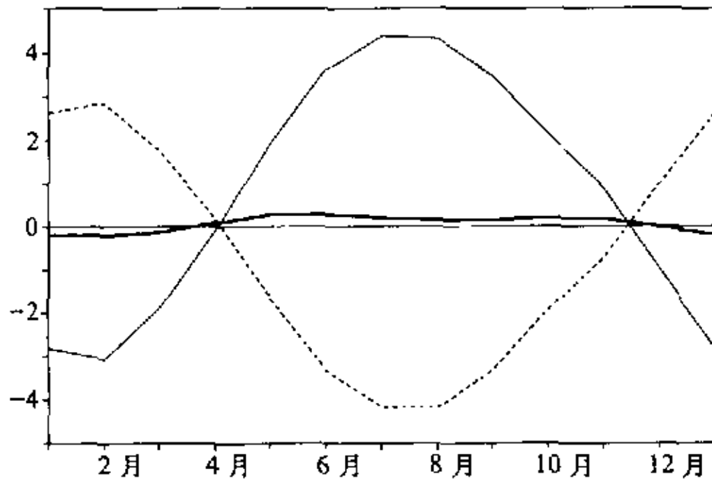
图 8 1958~1997 年赤道圈上指数 [\bar{I}] (粗实线)、 [\bar{I}_1] (虚线) 和 [\bar{I}_2] (细实线) 纬向平均的年变化 (单位: 10^3 \text{ kg m}^{-1} \text{ s}^{-1} )
