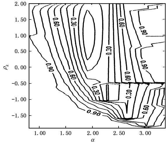
图 4 \left| \frac{\binom{k}{i}}{\binom{k}{j}} \right| < 1 的稳定区域等值线图
