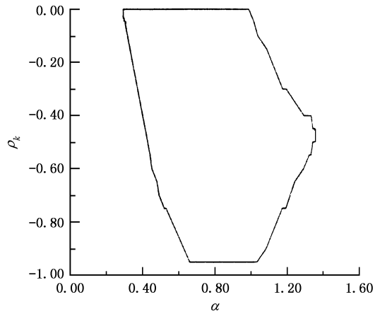
图2 |r_{1,k}| < 1 的稳定区域
